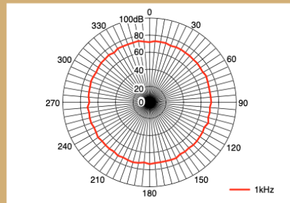
指向特性例
