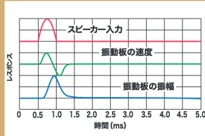
球形セラミックスコーカー fo:24kHz(実測値)
