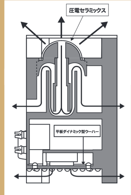
ES024 構造図
