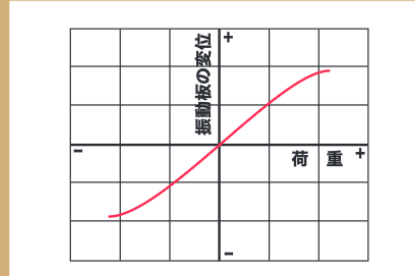
ウーハーの荷重vs.変位特性例
